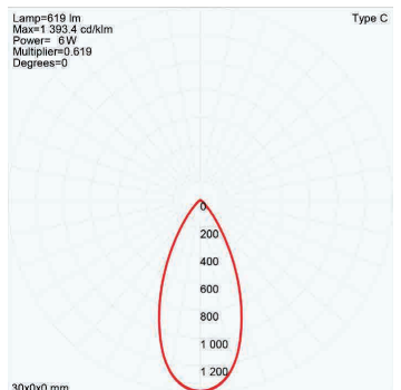
60° FWHM TIR
