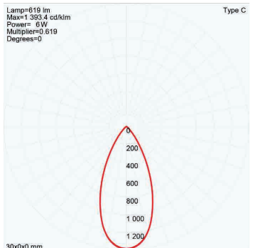
60° FWHM TIR
